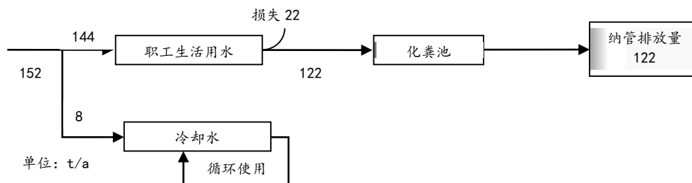
图 3-3 水平衡图
